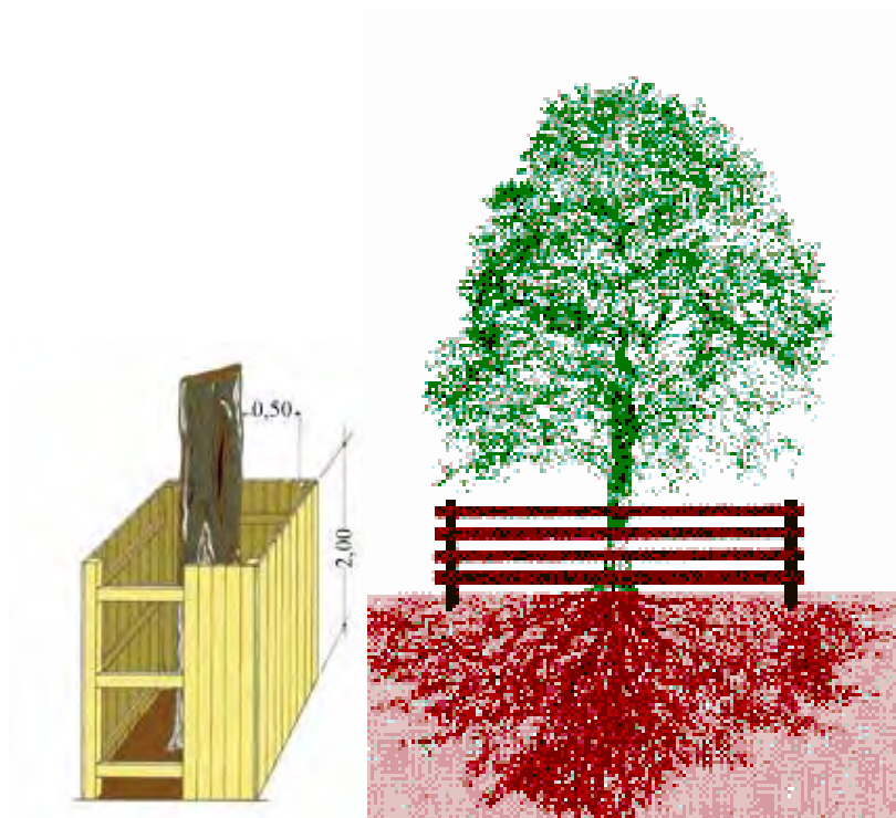
Illustration 2 : Exemples de protections en bois
