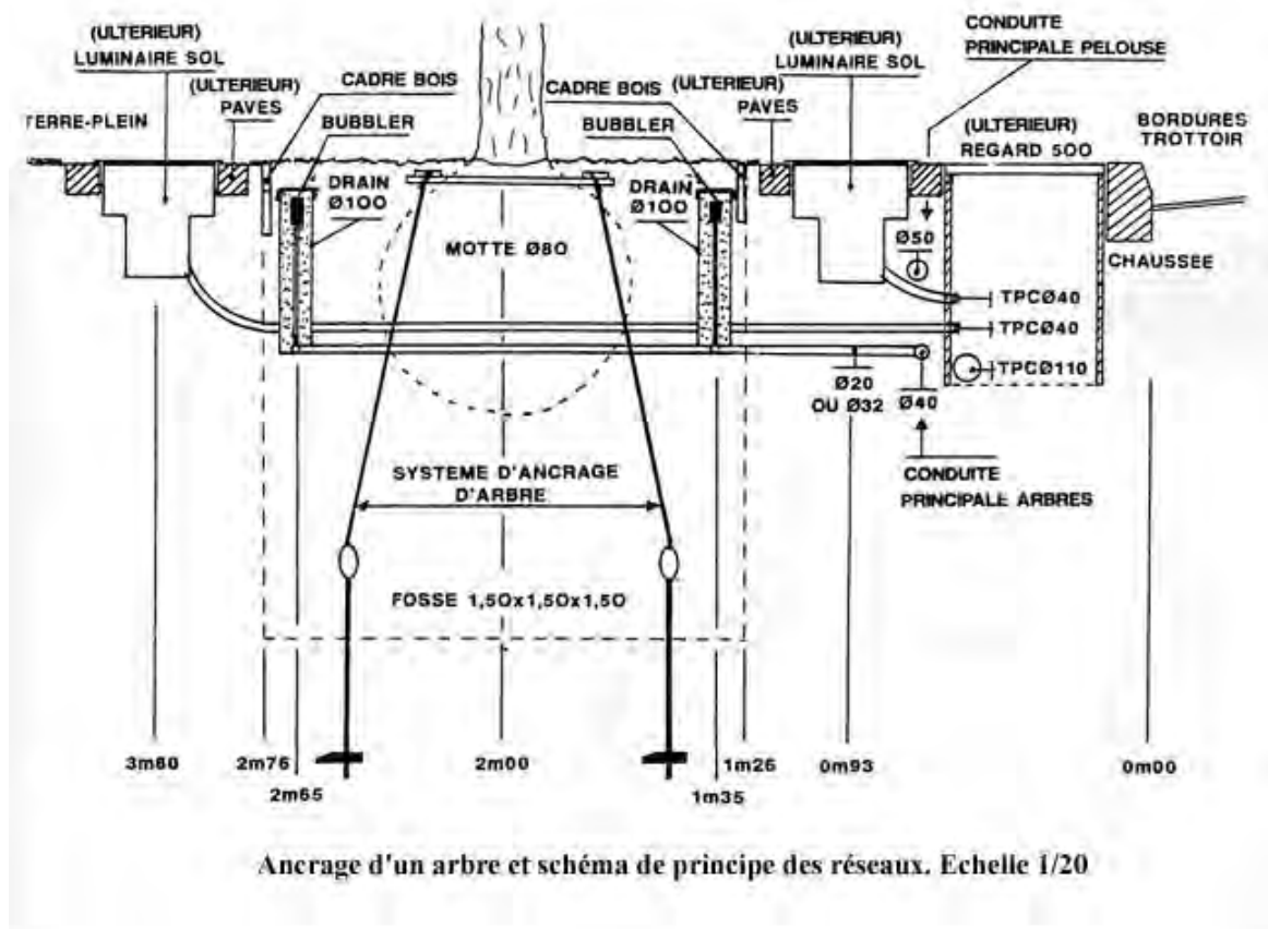
Illustration 19 : Ancrage
