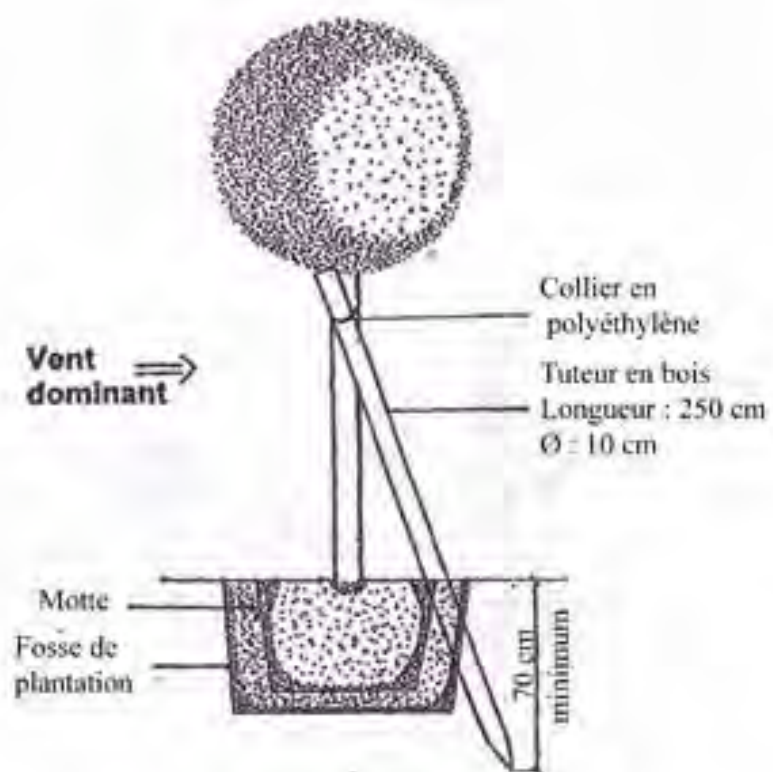
Illustration 17 : Tuteurage simple
